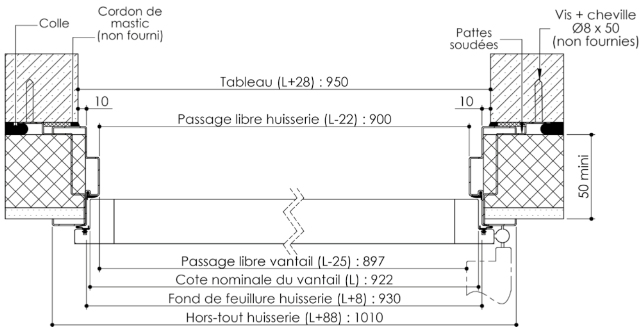
Seuil Alu PMR
