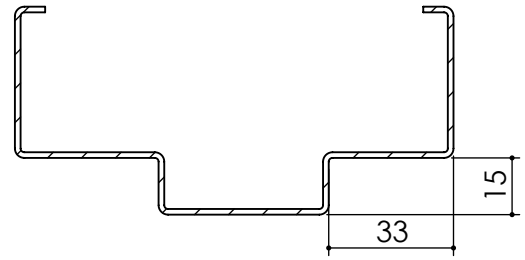
Huisserie non isophonique Pavillon service
