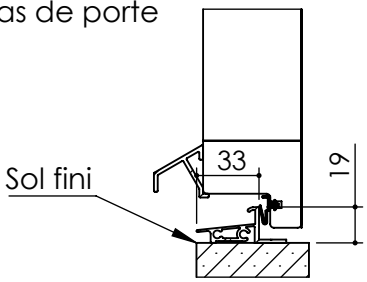
Seuil Alu PMR
