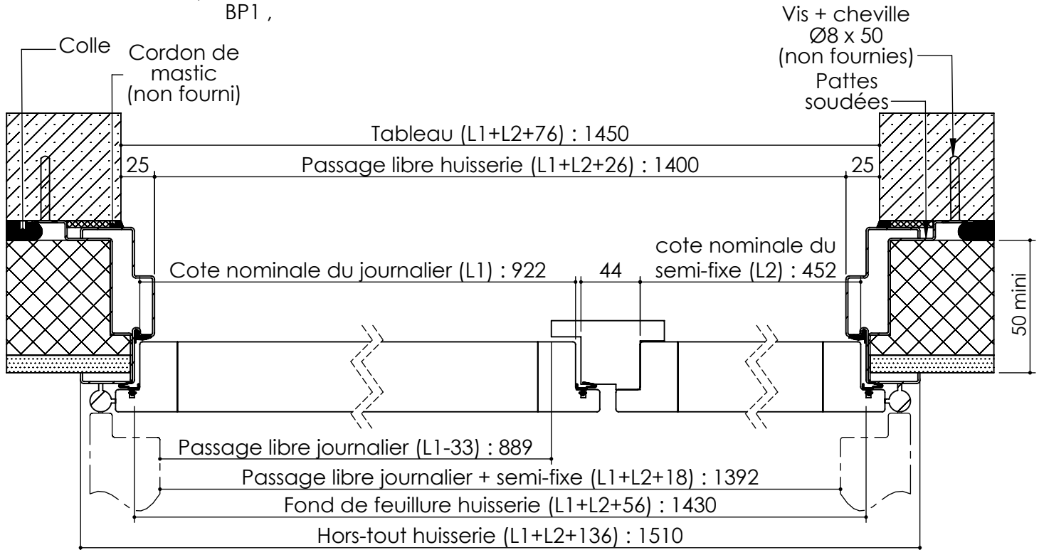
Huisserie non isophonique Pavillon service
