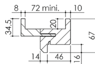
Huisserie isophonique
