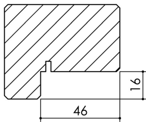
Huisserie isophonique
