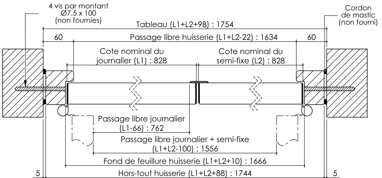
Huisserie isophonique
