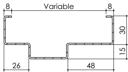
Huisserie non isophonique
