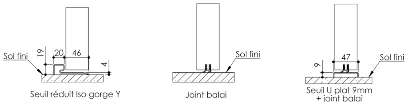
Variantes bas de portes
