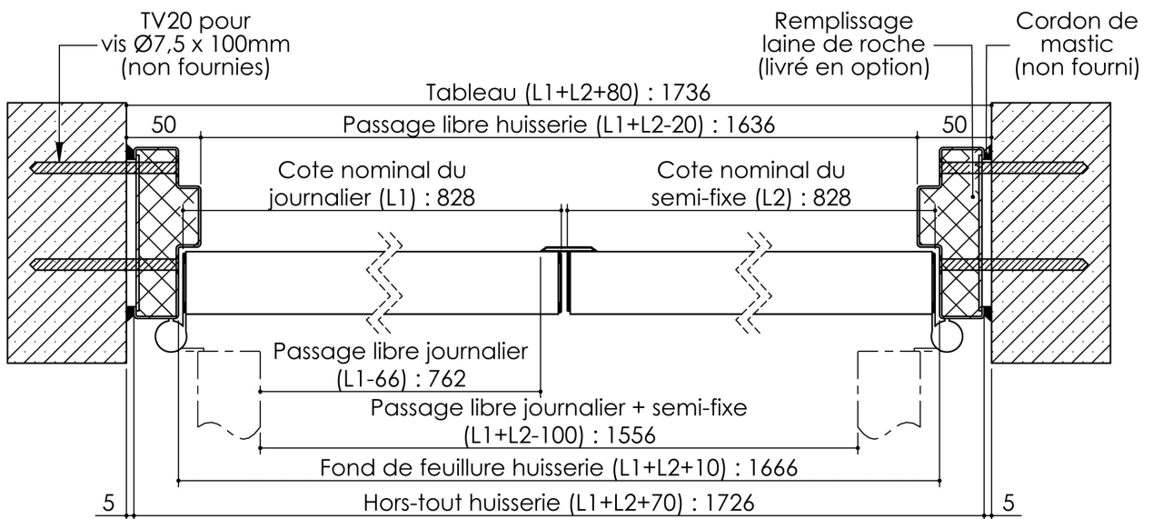
Huisserie isophonique
