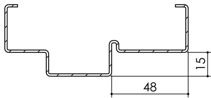
Huisserie isophonique
