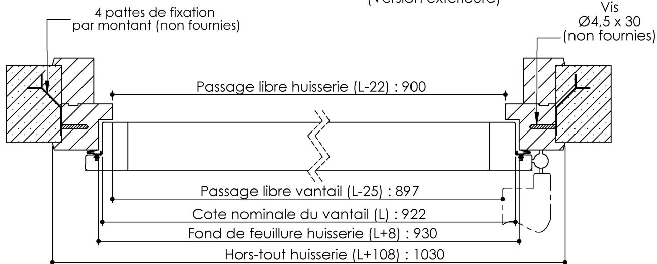
Option Seuil alu PMR (Version extérieure)
