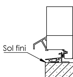
Option seuil alu PMR (Option extérieure)
